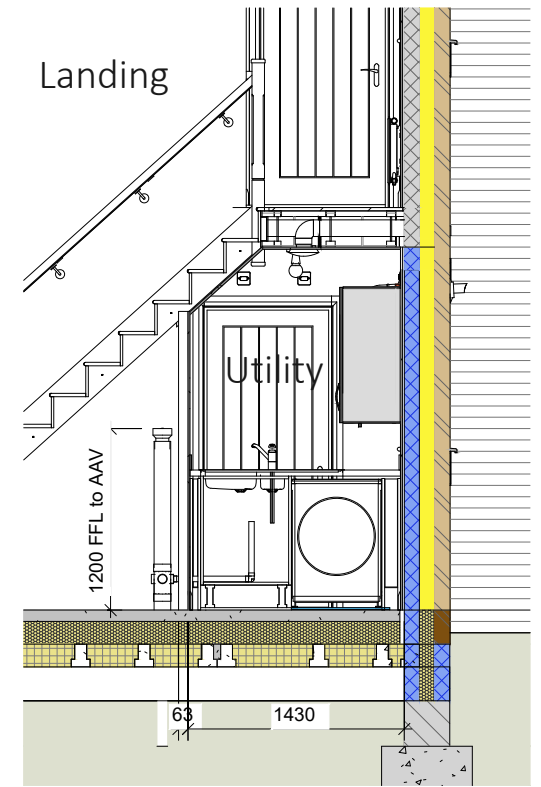
F Section F - F 1 : 50
